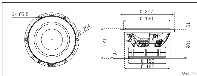
• Subwoofer 21 WX Be
