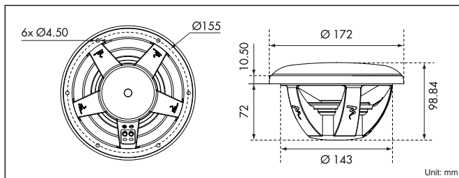
• Woofer 6 W3 Be - Kit N°7 & N°7 Active
