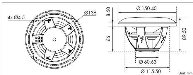
• Subwoofer 13 WS Be
