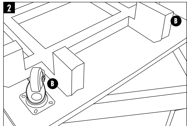
2 - Remove the cover of the box. - Unscrew the four wheels. 2 - Retirer le couvercle de la caisse. - Dévisser les 4 roulettes.
