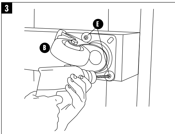
3 - Screw the wheels under the box with the supplied screws and collars. 3 - Visser les roues avec les vis et les rondelles fournies au dessous de la caisse.
